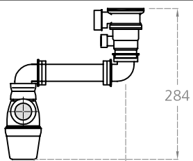
194 Trop Plein + Bonde à Tirette + Siphon Déplace réglable en hauteur 45<90
